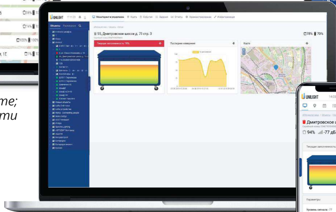
Интерфейс диспетчера
